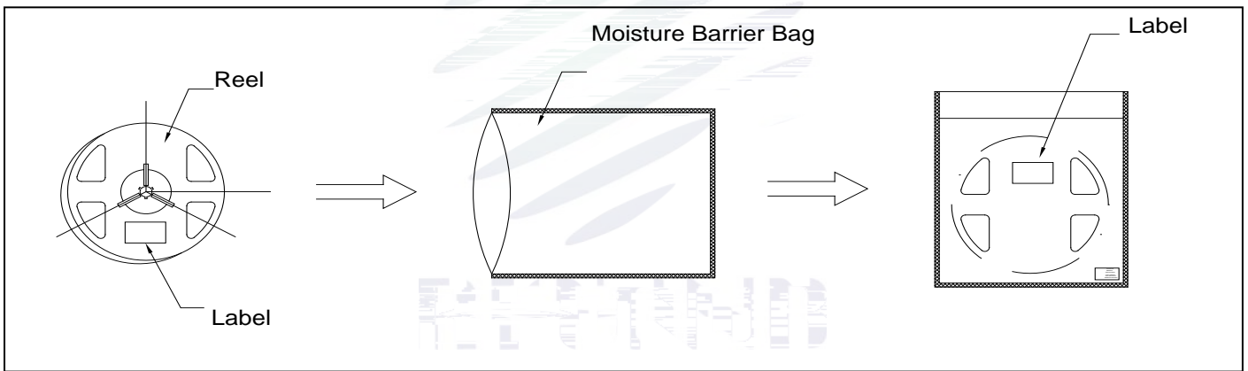
Fig.2-4 Moisture Resistant Packing eU? "-Xm
