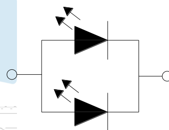
Fig.1-4 Polarity 极性
